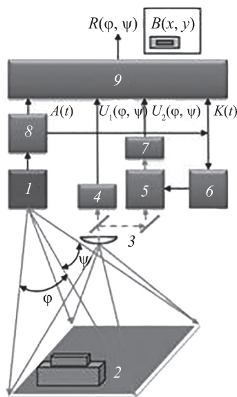
Рис. 1. Функциональная схема телевизионного лазерного локатора
