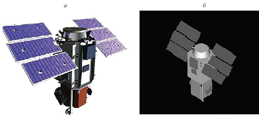
Рис. 6. Корпус исходного изображения космического аппарата (а) и его компьютерная трехмерная модель (б) (масштаб изготовленной модели объекта 1:100)
