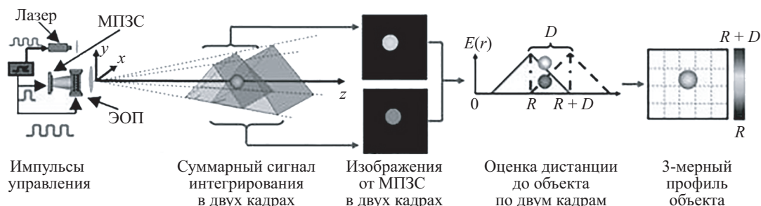
Рис. 3. Принцип работы многоимпульсной телевизионной системы для формирования трехмерного изображения
