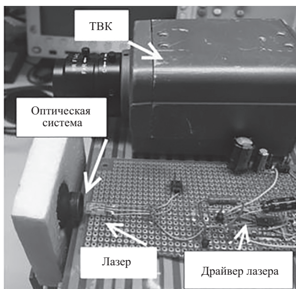
Рис. 4. Макет телевизионной лазерной системы
