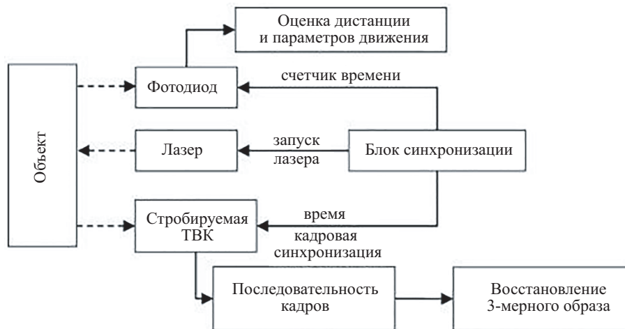
Рис. 2. Структурная схема flash-лидара
