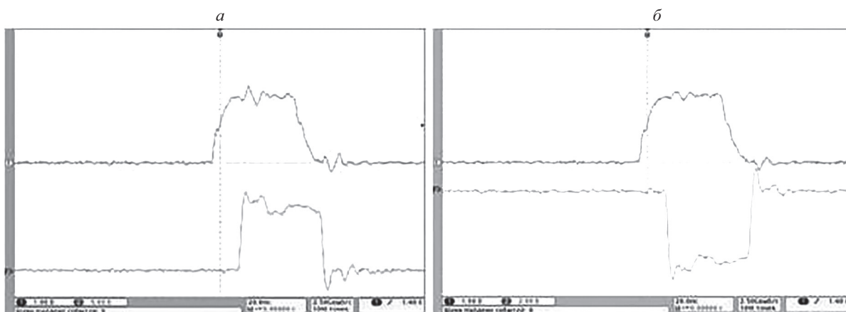
Рис. 5. Осциллограмма импульса управления лазером из камеры — верхняя (а), импульса лазера — нижняя (а), осциллограмма импульса накопления из камеры — верхняя (б), импульса накопления на входе прибора с зарядной связью — нижняя (б)
